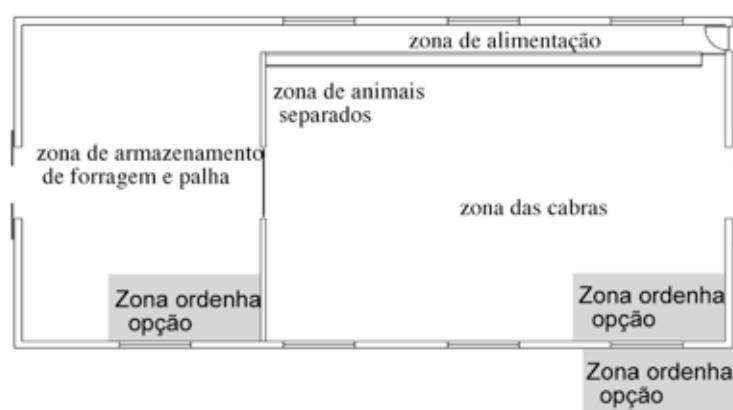
Figura 1- Alojamento com corredor de alimentação lateral.
